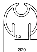
J 1188 0,241 Kg/m
