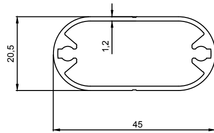
J 1056 0,490 Kg/m
