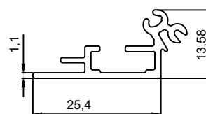
J 19123 0.222 Kg/m
