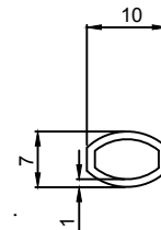
J 1242 0,068 Kg/m
