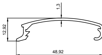
J 1181 0,275 Kg/m
