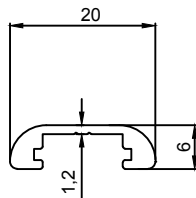
J 1509 0,140 Kg/m
