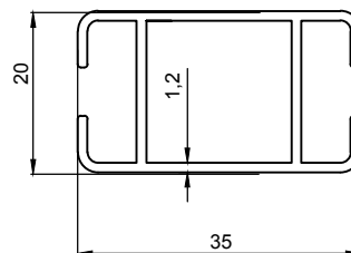
J 1185 0,405 Kg/m
