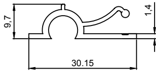
J 1173 0,221 Kg/m
